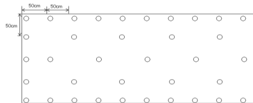
2.0m幅シートの場合
