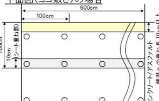
平面図(ヨコ敷きの場合)
