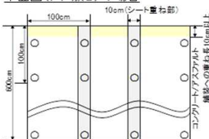
平面図(タテ敷きの場合)
