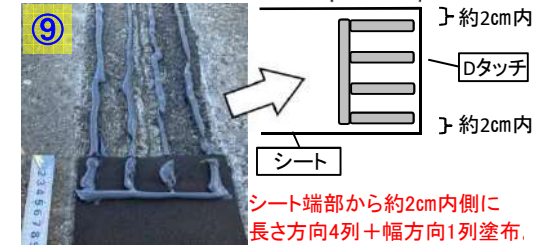
貼り付けたシートの表層にDタッチを塗布する。5cm以上重ねてシートを貼り付けた後ローラーで圧着し、Dタッチが均等にひろがるようにシート全体に馴染ませる。
