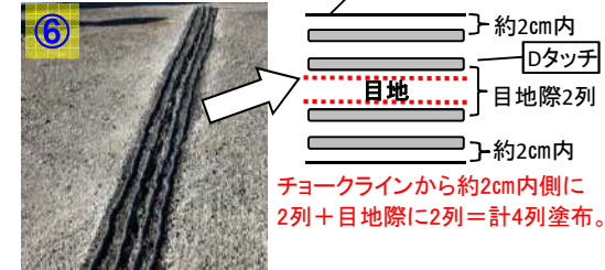
ノズルを先端から3番目でカットし、Dタッチを舗装面に4列塗布する。(1巻(5m)当り、Dタッチ3本使用目安) ※目地付近に段差がある場合は塗布方法を変更する。(2頁目参照)
