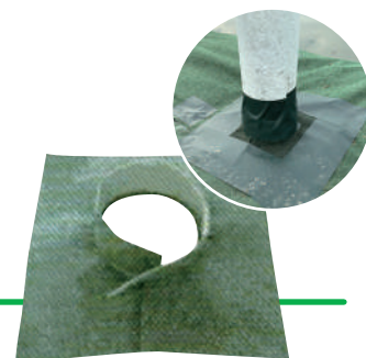
ガードレール支柱カバー
